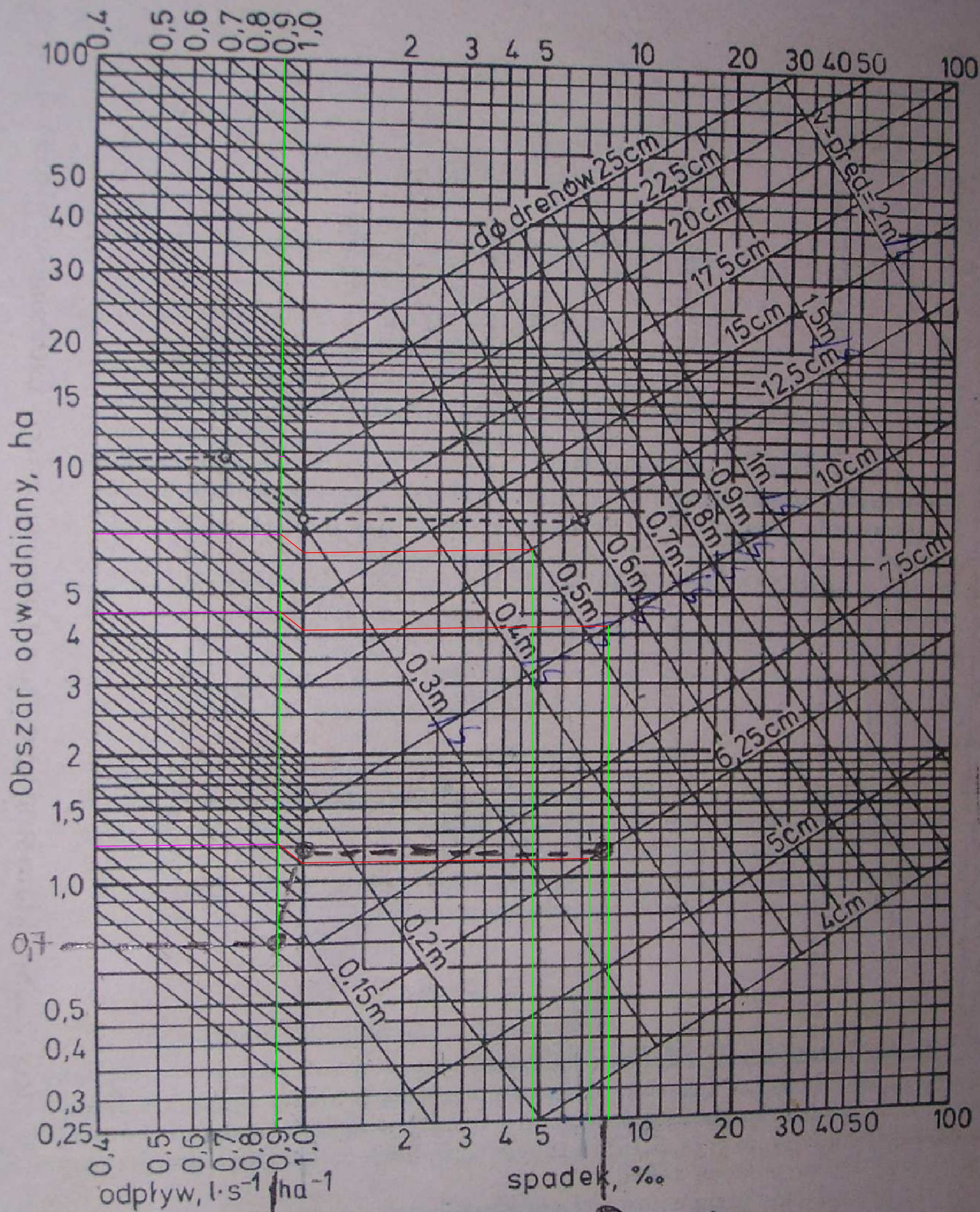
Rys. 5.153. Nomogram do określania średnic drenów ceramicznych
